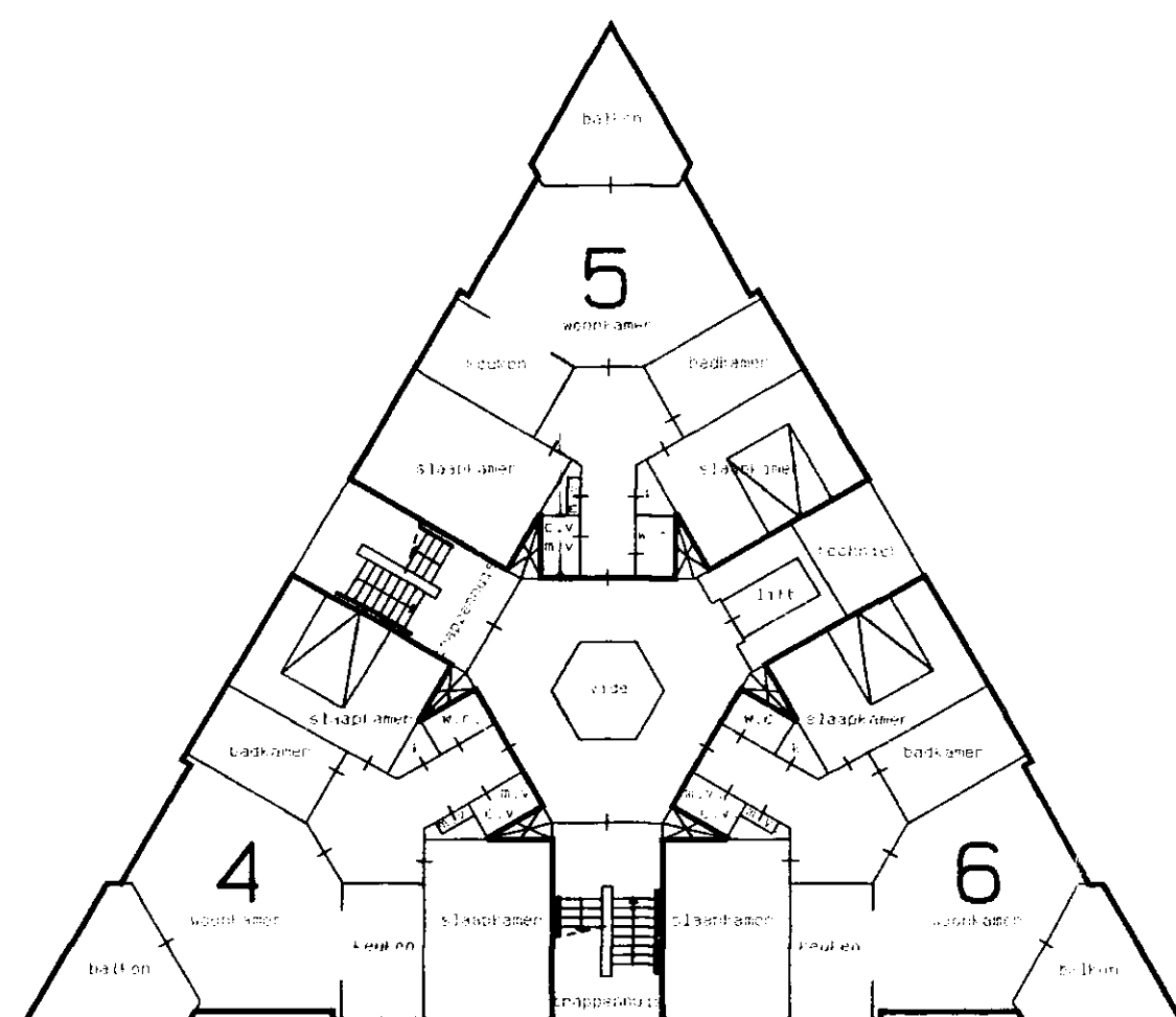
2e verdieping (schaal 1:200)
