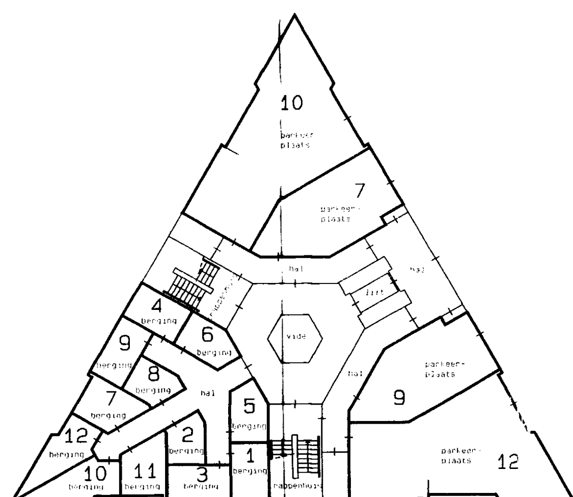
Beganegrond (schaal 1:200)
