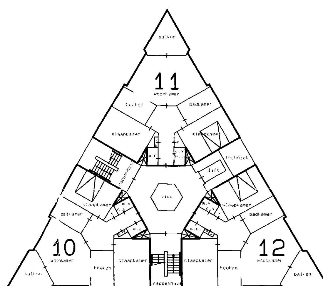
4e verdieping (schaal 1:200)
